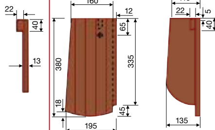
1 1/4 krawędziowa prawa Karpówka berlińska 19,5/38
