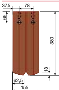
Półówka, podzielną Karpówka berlińska 15,5/38
